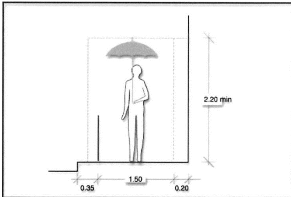
Σχήμα 1: Ελεύθερο ύψος
